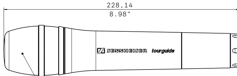
Mikrofonkopf microphon basket
