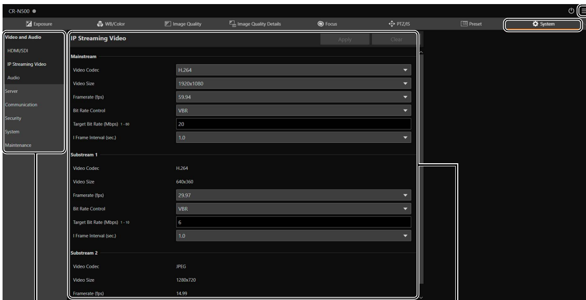
Einstellungselementkategorie
